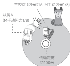
使用一个从属灯进行无线闪光拍摄
