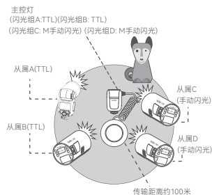
使用四个从属灯进行无线闪光拍摄
